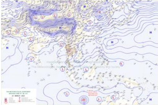
แผนที่อากาศผิวพื้น วันที่ 25 มีนาคม 2568 เวลา 07:00
