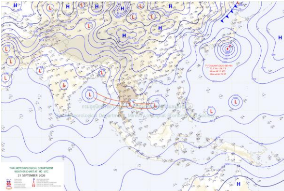
แผนที่อากาศผิวพื้น วันที่ 21 กันยายน 2569 เวลา 07:00 น.
